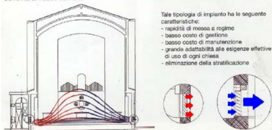
Schema di flusso dell'aria
