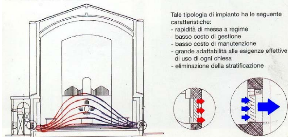
Schema di flusso dell'aria
