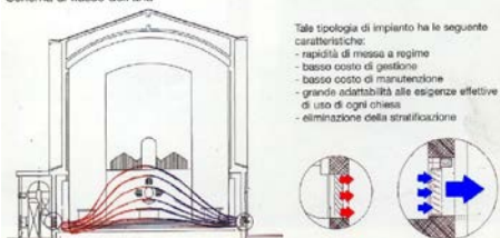
Schema di flusso dell'aria
